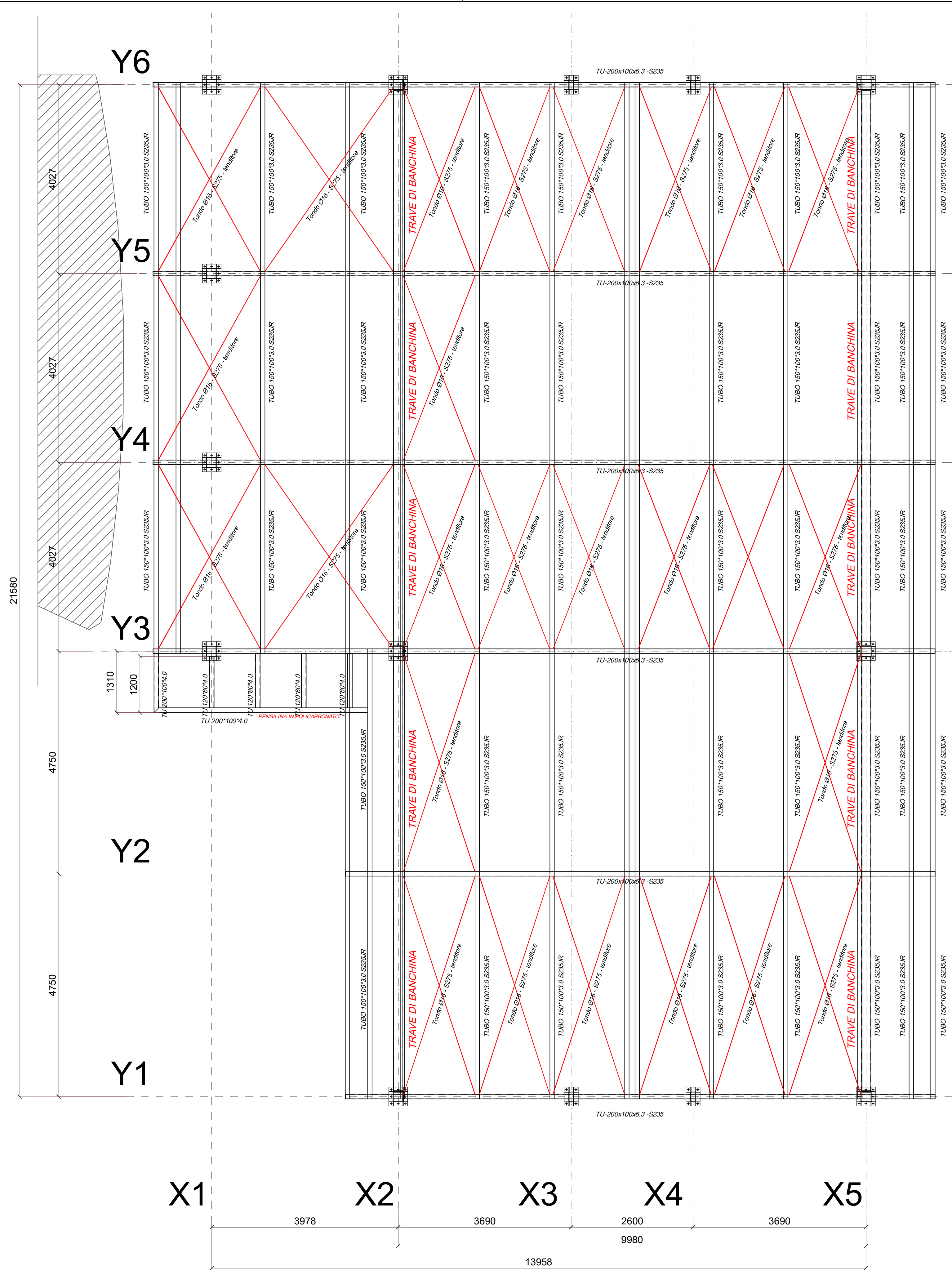
Pianta della copertura Scala 1:50
